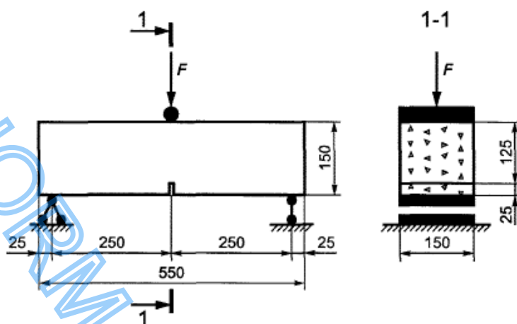
Рисунок Б.1 - Схема испытания образца
