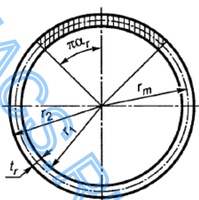
Рисунок 6 - Схема кольцевого сечения сталефибробетонного элемента, принимаемая при его расчете по прочности на изгиб
