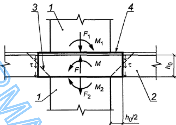
1 - колонна; 2 - плита; 3 - пирамида продавливания; 4 - условный расчетный контур
