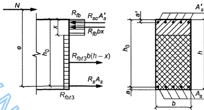
Рисунок 9 - Схема усилий и эпюра напряжений в сечении, нормальном к продольной оси внецентренно сжатого сталефибробетонного элемента с рабочей арматурой, при расчете ее по прочности
