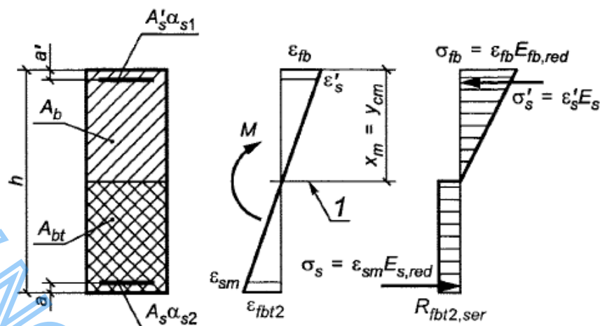
1 - уровень центра тяжести поперечного сечения
