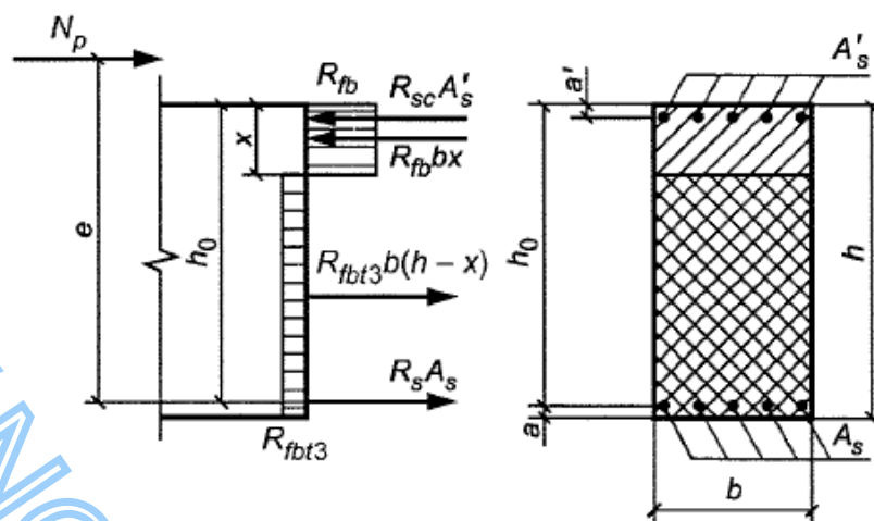
Рисунок 22 - Схема усилий и эпюра напряжений в сечении, нормальном к продольной оси изгибаемого предварительно напряженного элемента при его расчете по прочности в стадии обжатия
