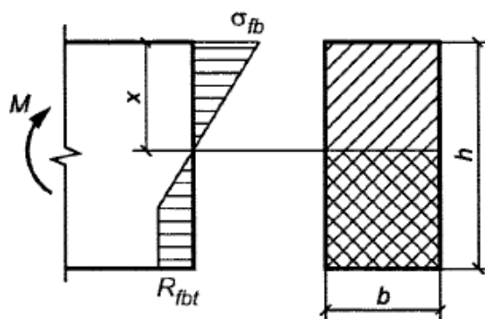
Рисунок 2 - Схема усилий и эпюра напряжений в сечении, нормальном к продольной оси изгибаемого сталефибробетонного элемента прямоугольного сечения без арматуры при его расчете по прочности
